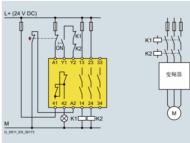
常规接线
