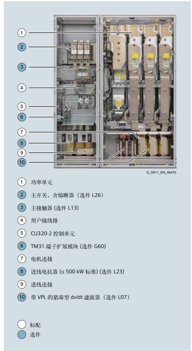
示例：SINAMICS G150 变频调速柜的结构，A 型
